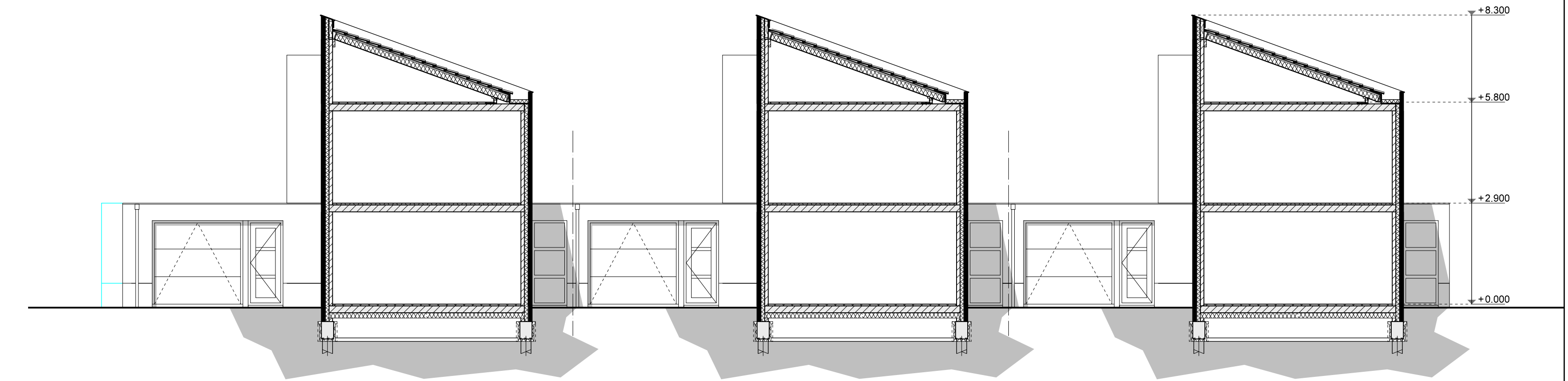
Dwarsdoorsnede A-A
